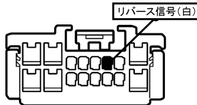
①ヒューズボックス内コネクタ16P(緑)
