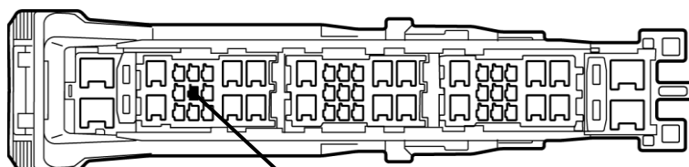
①ヒューズボックス内コネクタ49P(緑)
