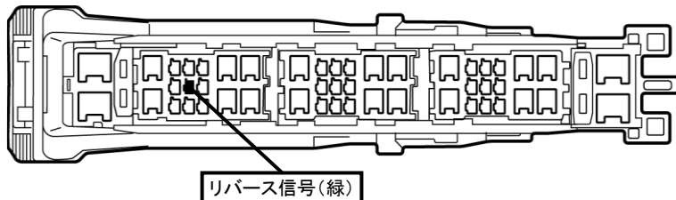
①ヒューズボックス内コネクタ49P(緑)
