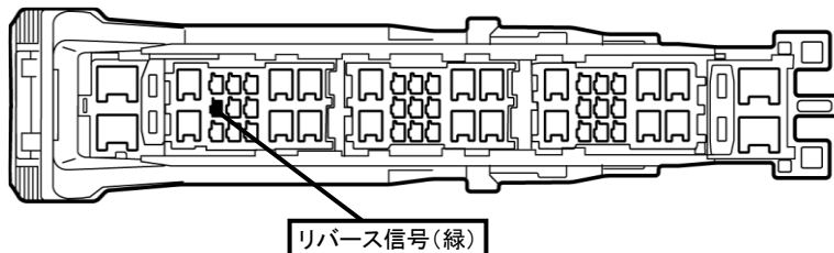
②ヒューズボックス内コネクタ49P(緑)
