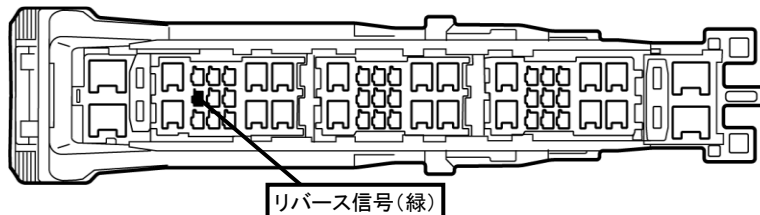
ヒューズボックス内49Pコネクタ(緑)
