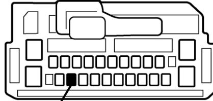
車速信号(灰)
