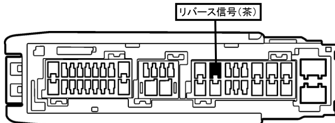
ヒューズボックス内コネクタ42P(緑)
