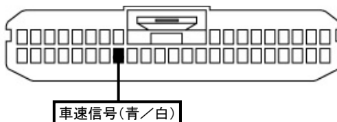
①メーターユニット40Pコネクタ(白)
